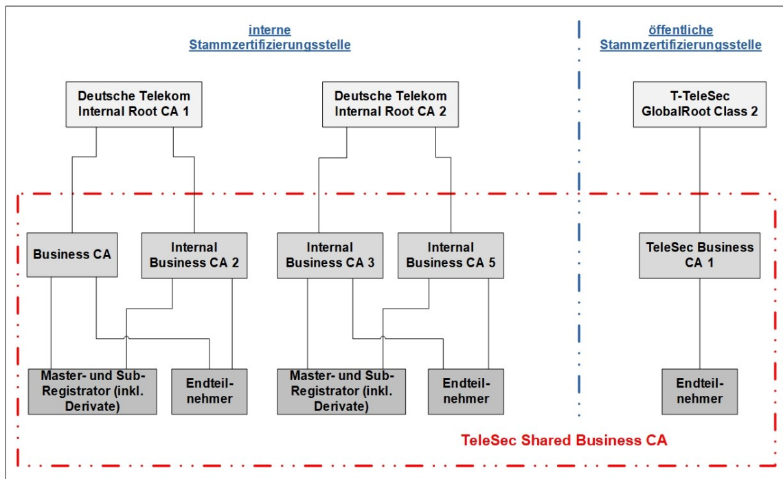
Abbildung 1: Übersicht der PKI-Dienstleistung „TeleSec Shared-Business-CA“ mit den jeweiligen Root- und Sub-CAs
