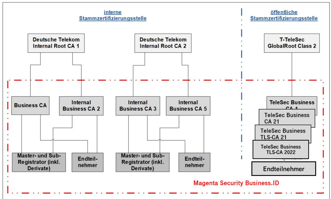
Abbildung 1: Übersicht der PKI-Dienstleistung „Business.ID“ mit den jeweiligen Stamm- und Zwischenzertifizierungsstellen (Root- und Intermediate-CAs, Sub-CAs)
